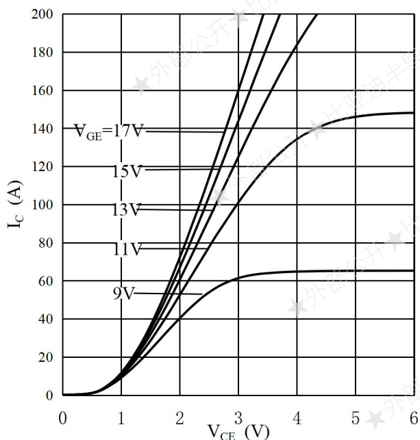
图 3 输出特性
