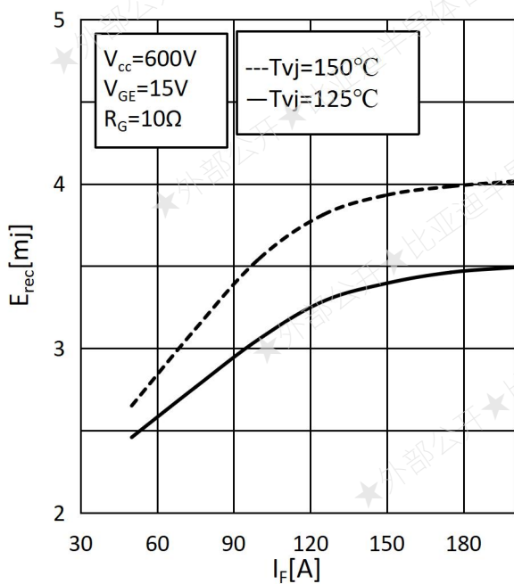
图 7 开关损耗二极管-逆变器 Fig.7 Typ. Switching Losses Diode-Inverter
