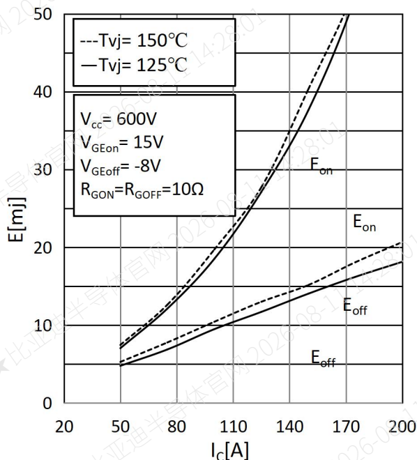
图 4 开关损耗和集电极电流
