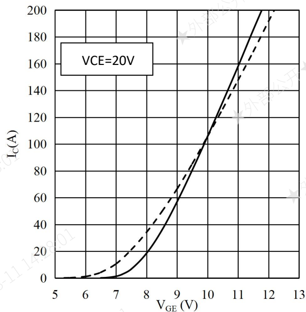
图 2 传输特性
