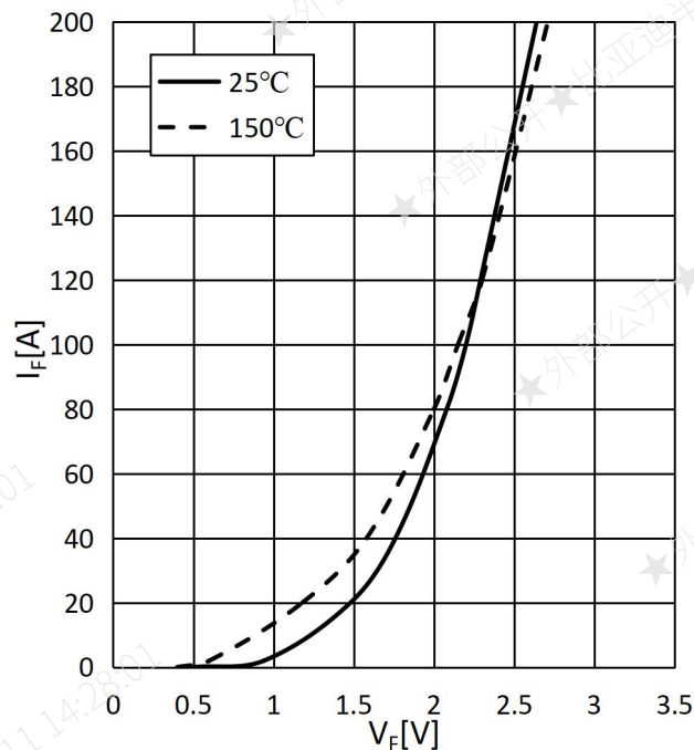
图 6 二极管输出特性 Fig.6 FWD Forward Characteristics
