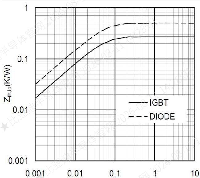
图 9 瞬态热阻
