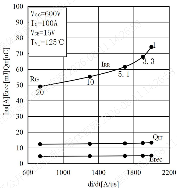
图 5 反向恢复特性和 di/dt
