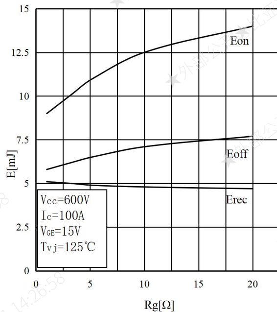
图 6 开关损耗和门极电阻
