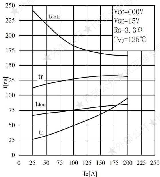
图 7 开关时间和集电极电流
