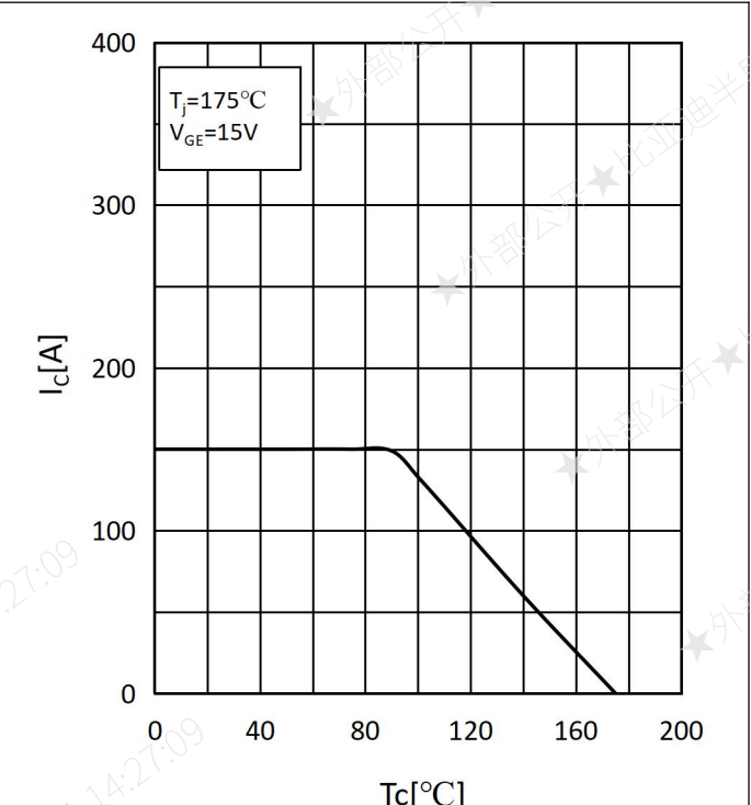
Fig. 10 Rate Current vs. Temperature (Tc) 图 10 额定电流和温度
