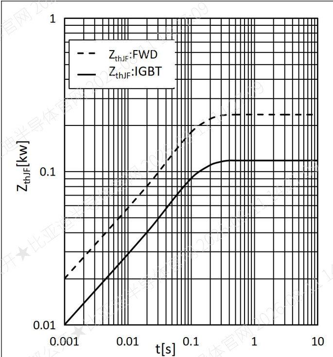
Fig.9 Typ. Transient Thermal Impedance 图 9 瞬态热阻
