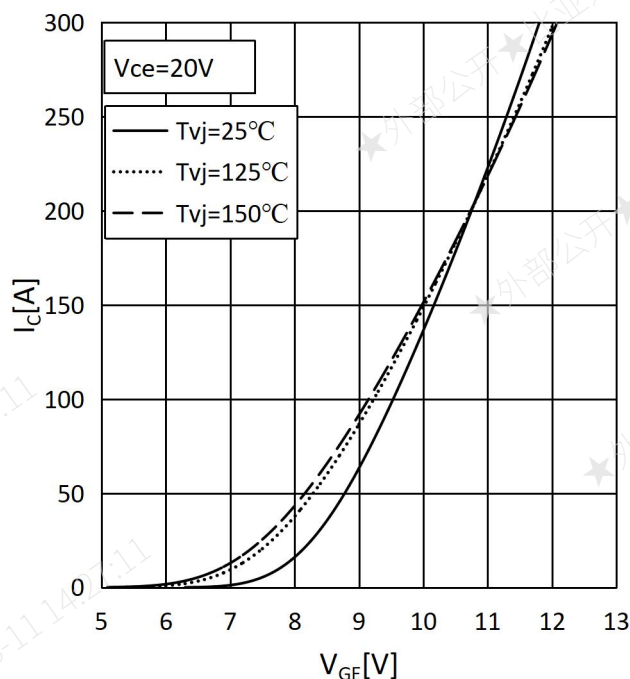
图 2 传输特性
