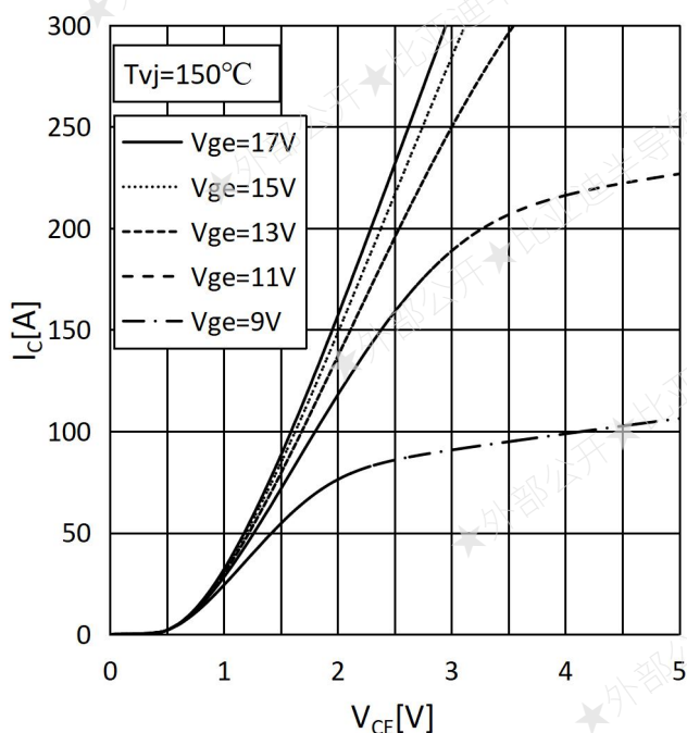
图 3 输出特性
