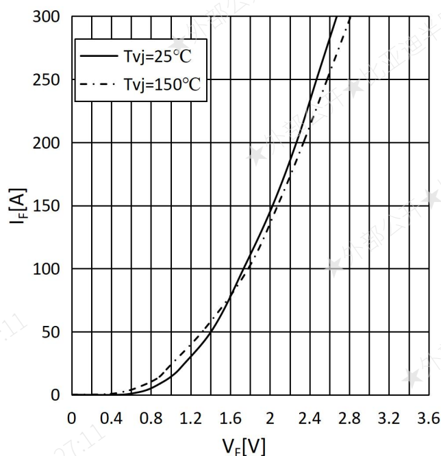
图 6 二极管输出特性
