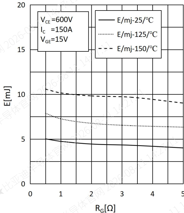
图 8: 反向恢复损耗与门极电阻关系
