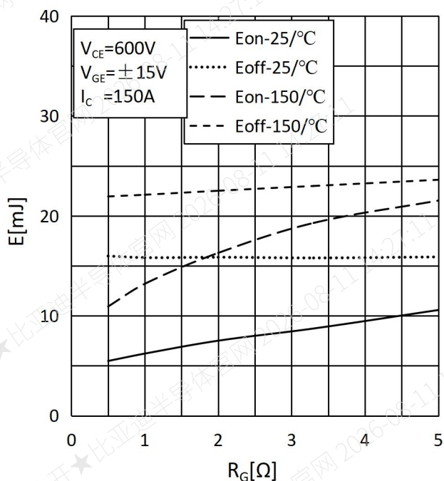
图 5 开关损耗和门极电阻
