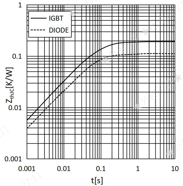
图 10 瞬态热阻
