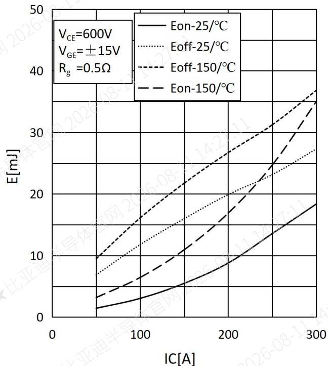
图 4 开关损耗和集电极电流
