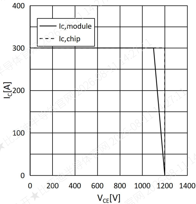
图 9 反偏安全工作区
