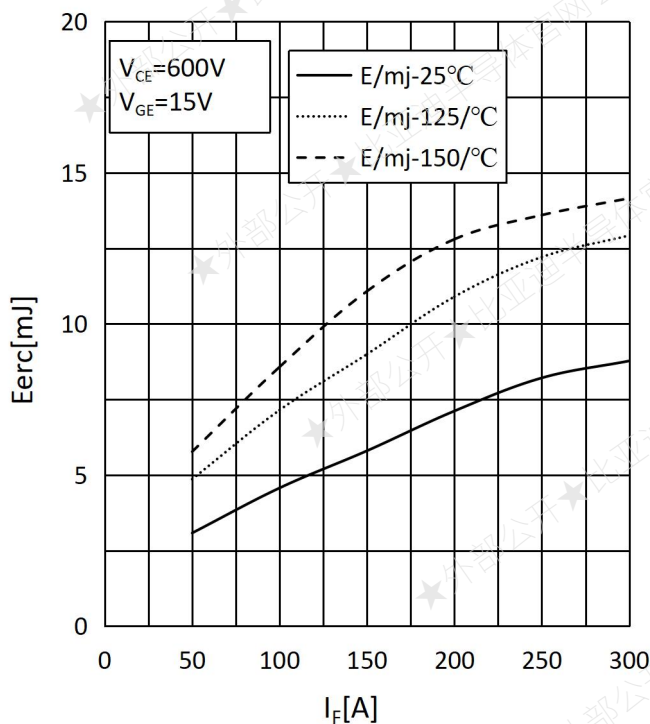
图 7 反向恢复损耗
