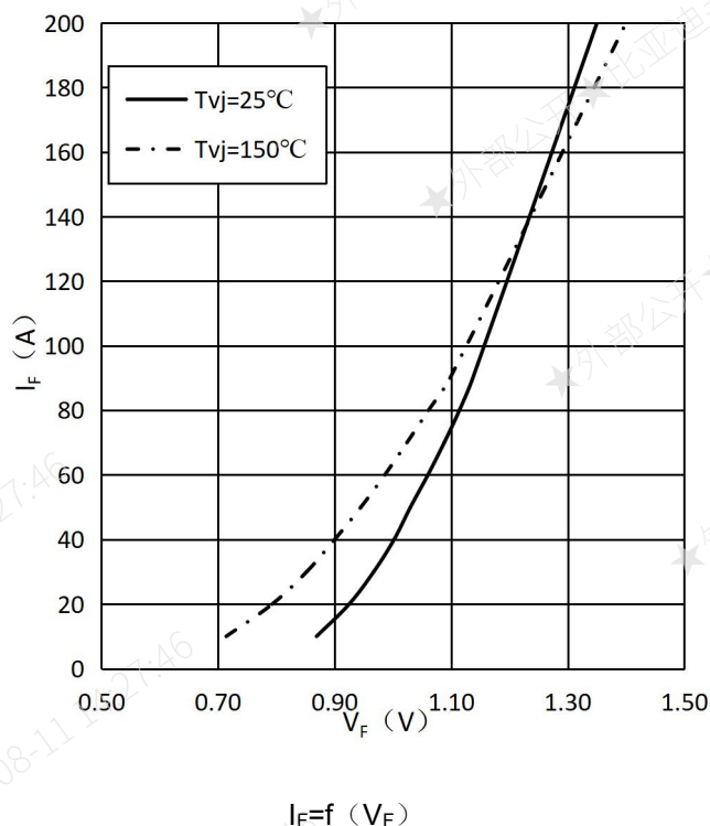
Fig.10 Forward Characteristics of Diode-Rectifier 图 10 二极管正向偏压特性-整流器
