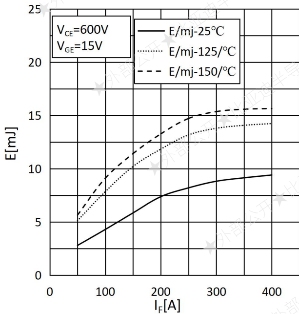
图 7 反向恢复损耗
