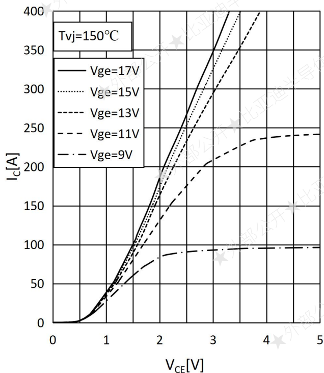
图 3 输出特性
