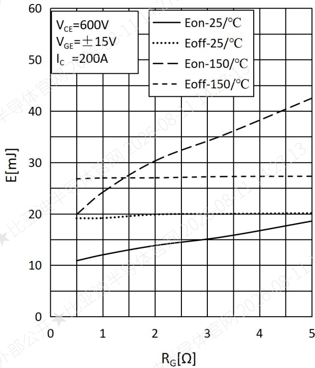
图 5 开关损耗和门极电阻
