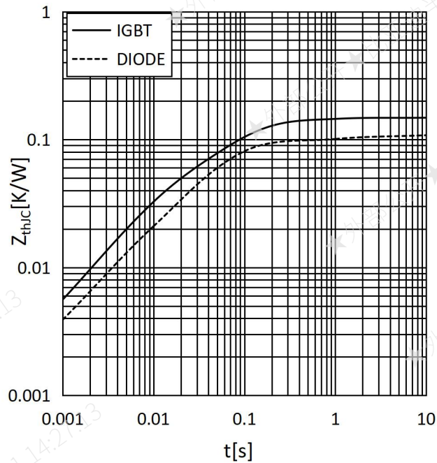
图 10 瞬态热阻
