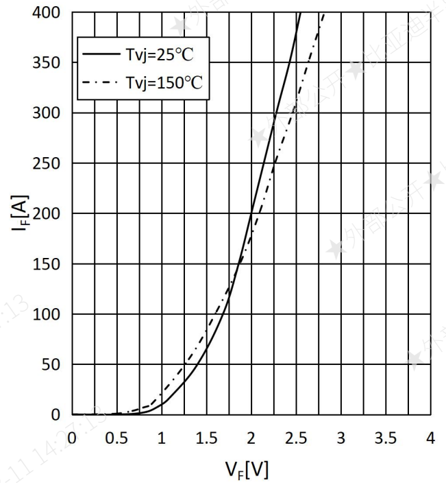
图 6 二极管输出特性
