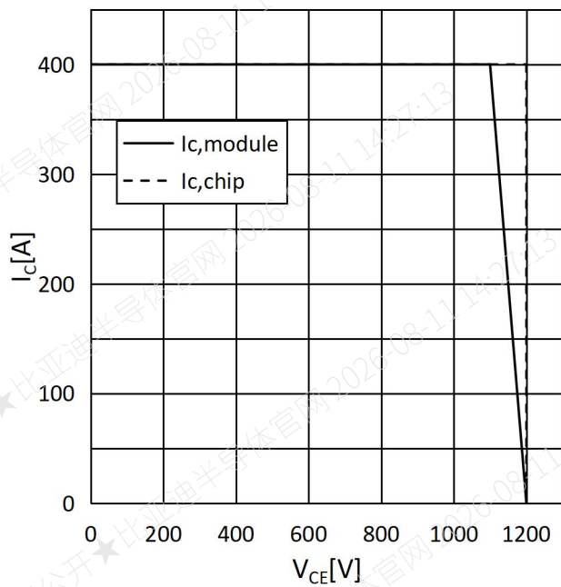
图 9 反偏安全工作区
