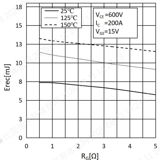
图 8: 反向恢复损耗与门极电阻关系
