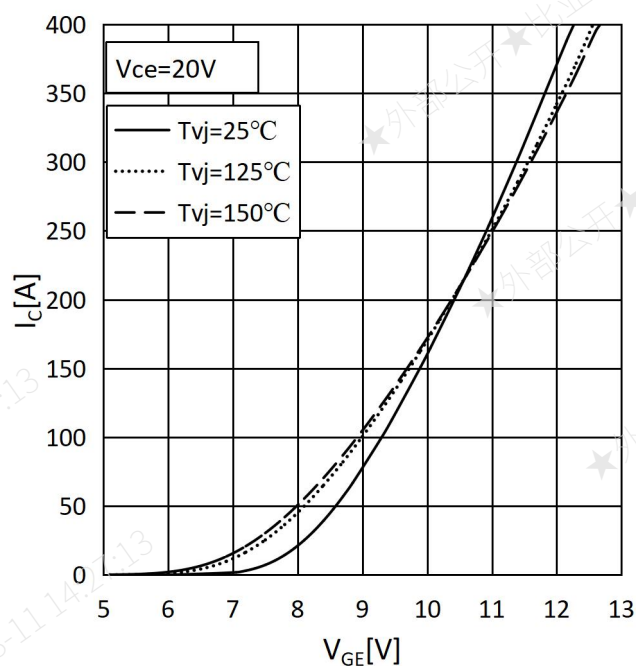
图 2 传输特性
