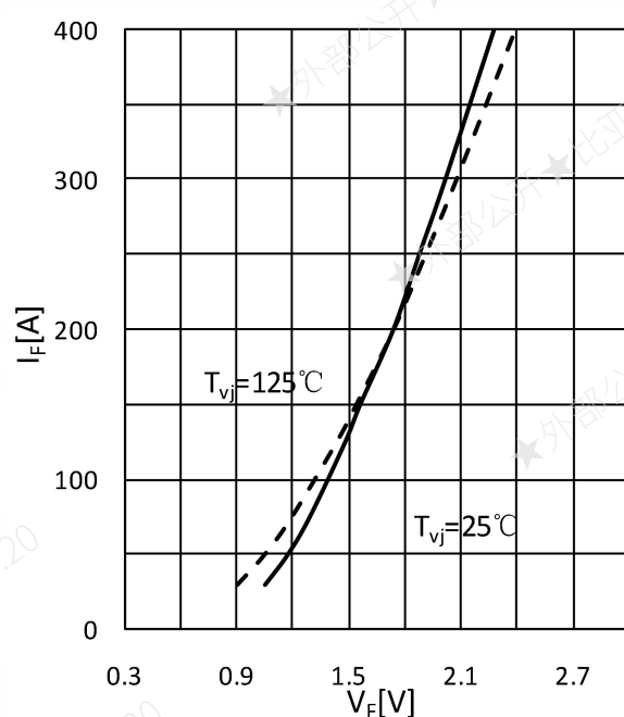
Fig.6 FWD Forward Characteristics 图 6 二极管输出特性
