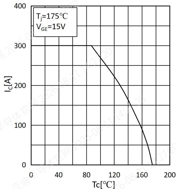
Fig.8 Rate Current vs. Temperature ( T_c ) 图 8 额定电流和温度
