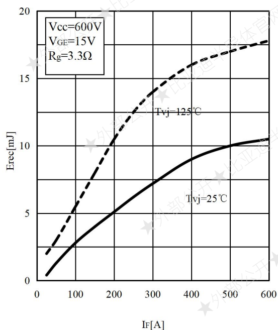
Fig.7 Typ. Switching Losses Diode-Inverter 图 7 开关损耗二极管-逆变器
