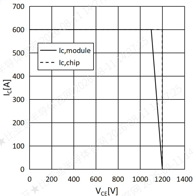
图 9 反偏安全工作区
