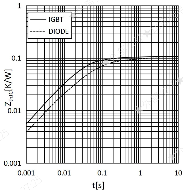
图 10 瞬态热阻
