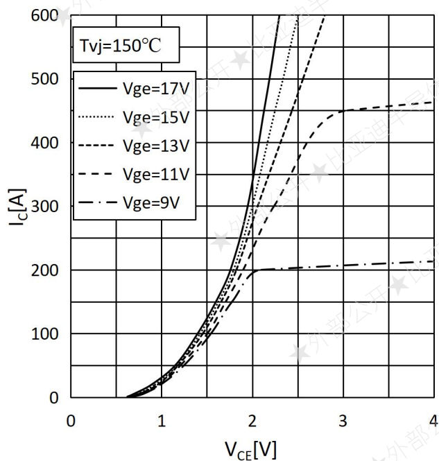
图 3 输出特性
