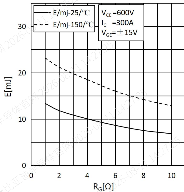
图 8: 反向恢复损耗与门极电阻关系
