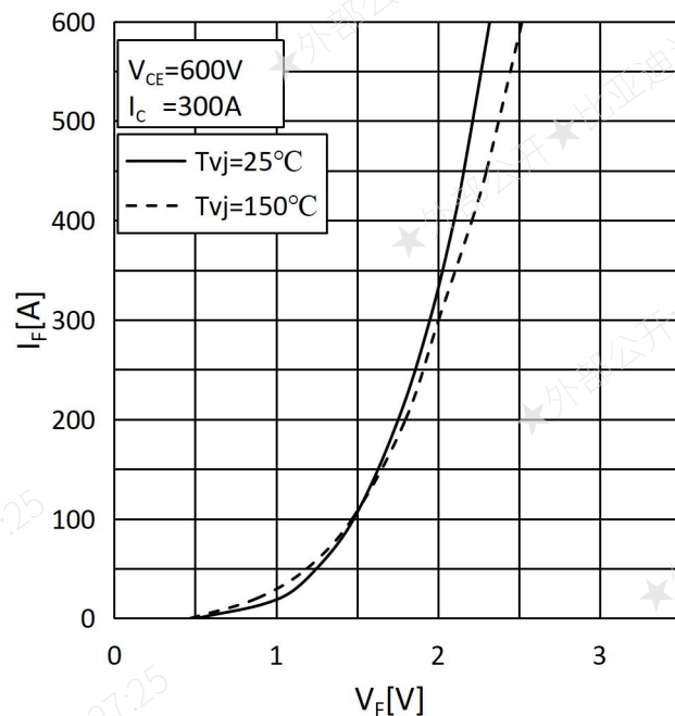
图 6 二极管输出特性
