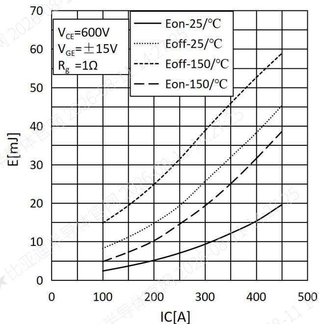
图 4 开关损耗和集电极电流
