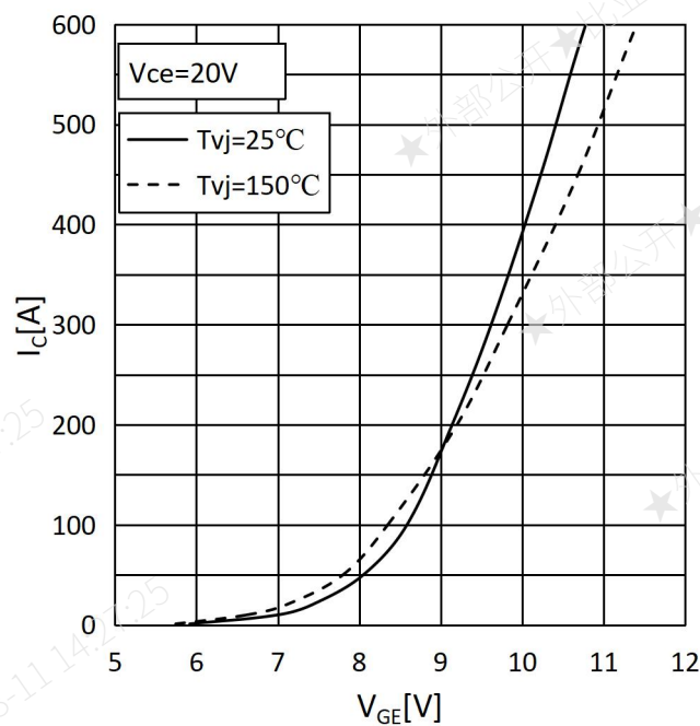
图 2 传输特性
