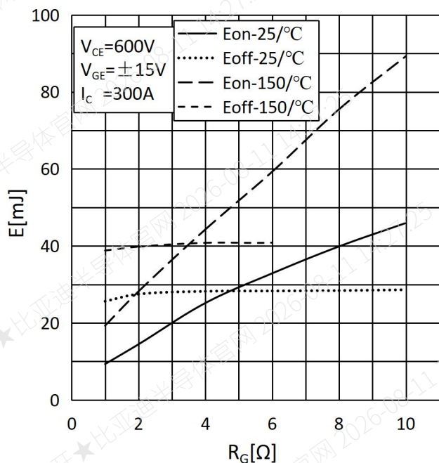
图 5 开关损耗和门极电阻
