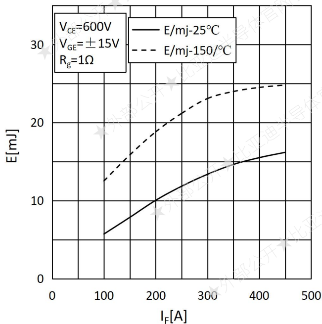
图 7 反向恢复损耗
