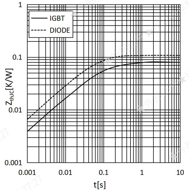
图 10 瞬态热阻
