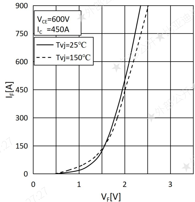
图 6 二极管输出特性 Fig.6 FWD Forward Characteristics
