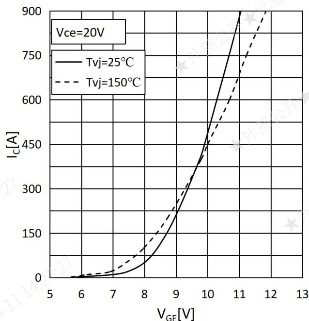
图 2 传输特性
