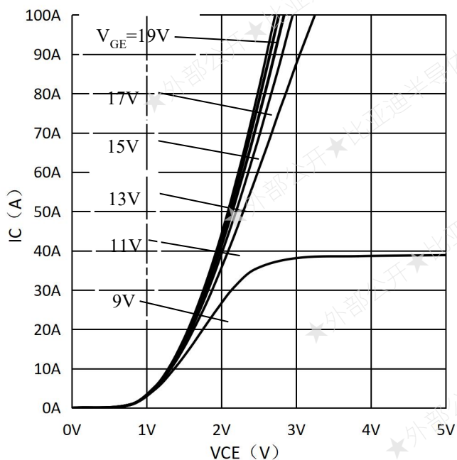
图 1 输出特性-逆变器
