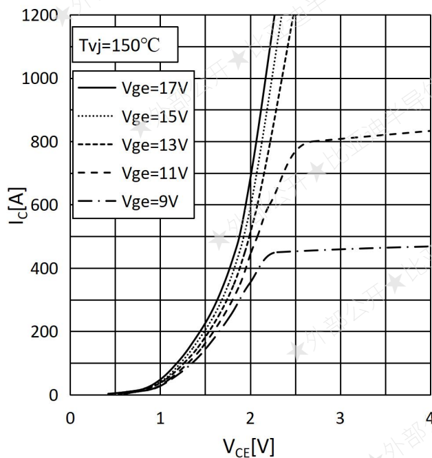
图 3 输出特性
