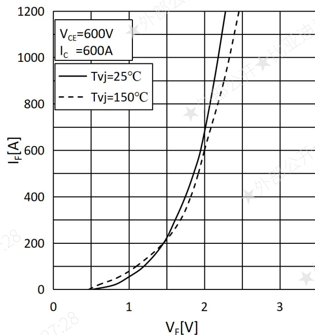
图 6 二极管输出特性
