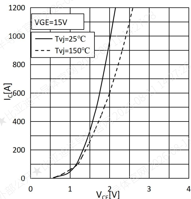
图 1 开通状态特性
