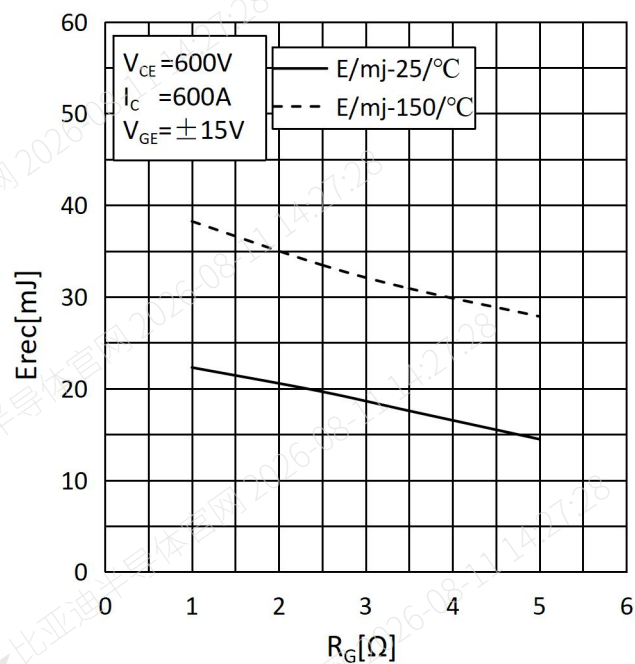
图 8: 反向恢复损耗与门极电阻关系
