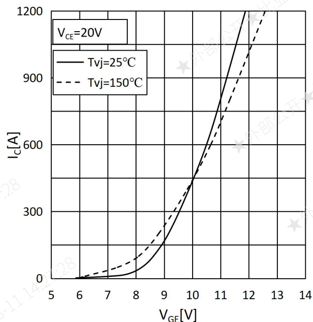
图 2 传输特性
