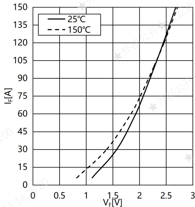
图 6 二极管输出特性 Fig.6 FWD Forward Characteristics
