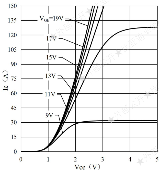
图 3 输出特性
