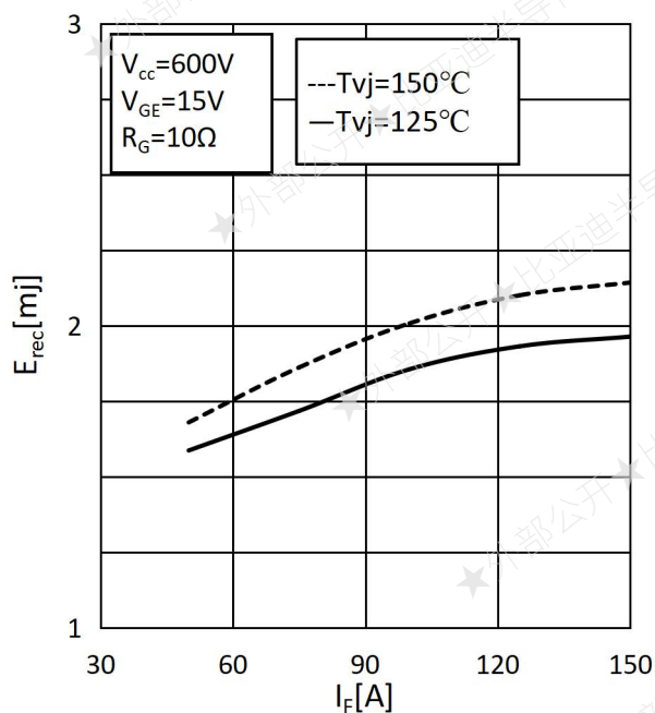
图 7 开关损耗二极管-逆变器 Fig.7 Typ. Switching Losses Diode-Inverter
