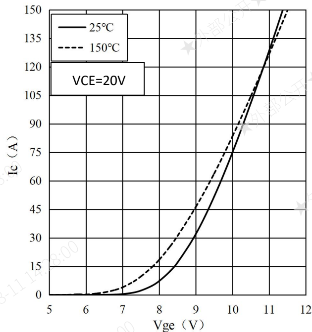
图 2 传输特性
