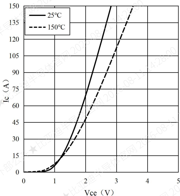
图 1 开通状态特性
