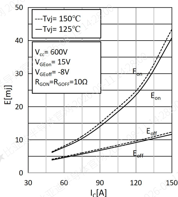
图 4 开关损耗和集电极电流
