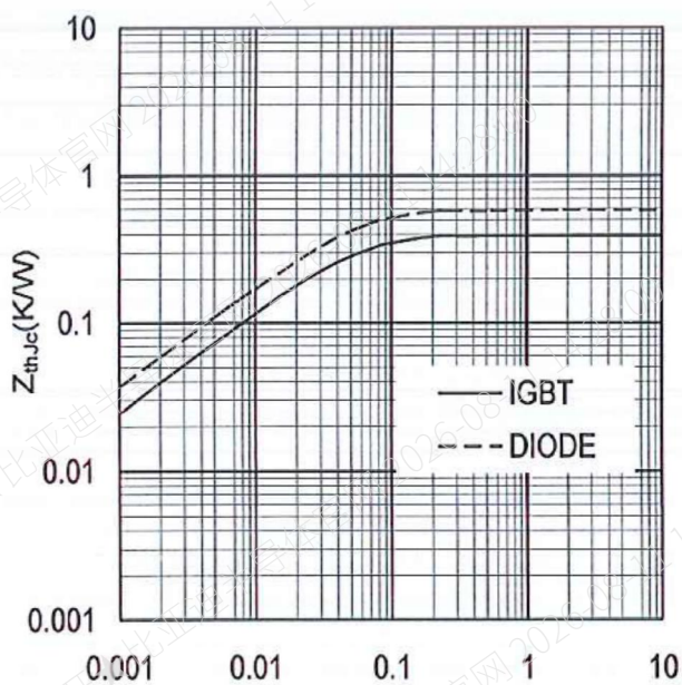
图 9 瞬态热阻
