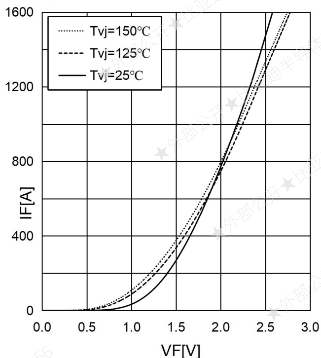
Fig.7: Forward characteristic 图 7: 正向特性
