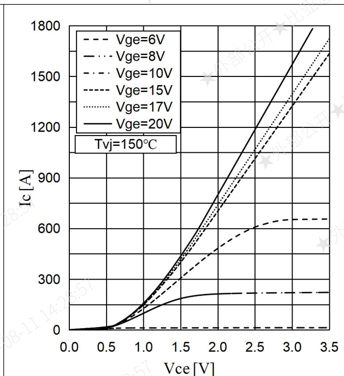
Fig.2: Output Characteristics 图 2: 输出特性
