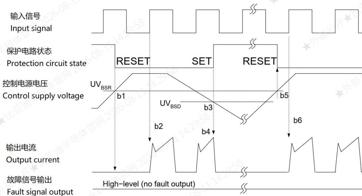
图 7. 高边欠压保护
