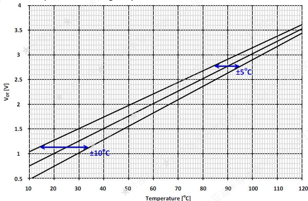
图 5. 温度输出电压
