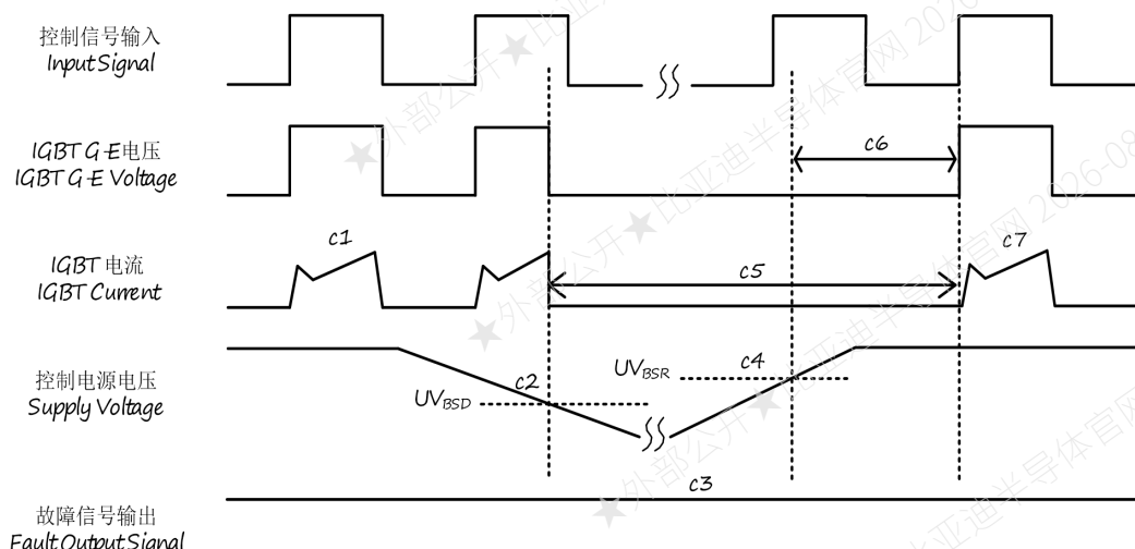
图 9.上桥欠压保护
