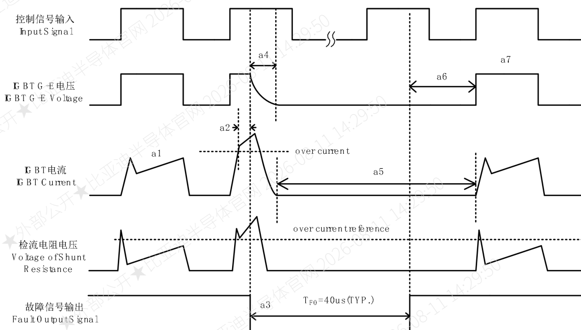
图 7.过流保护
