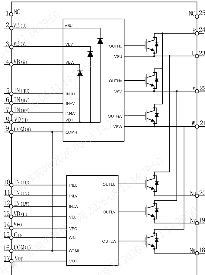
图1. 内部等效电路 Fig 1. Internal Equivalent Circuit
