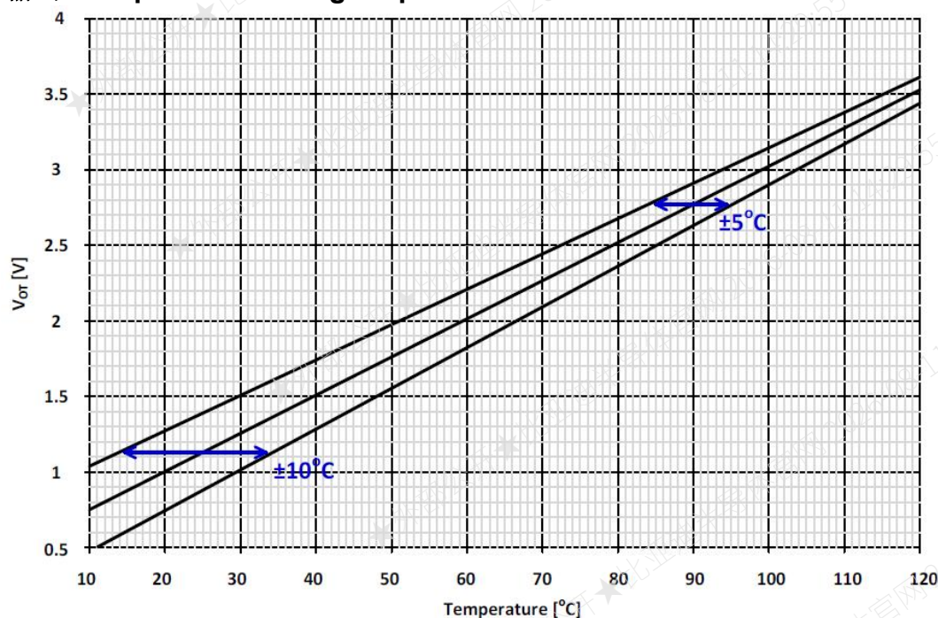
图 5. 温度输出电压 Fig 5. Voltage of temperature
