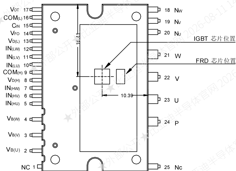
图 2. 引脚布局图(top view)
