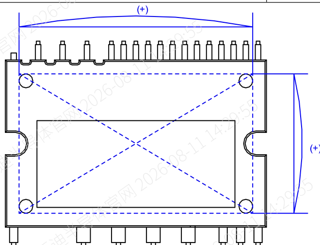
图 6. 平面度测量位置 Fig 6. Flatness Measurement Position
