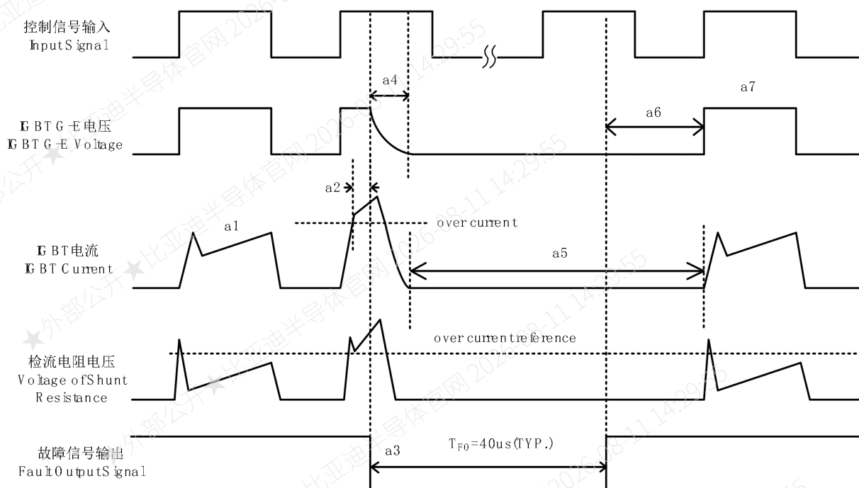
图 7.过流保护
