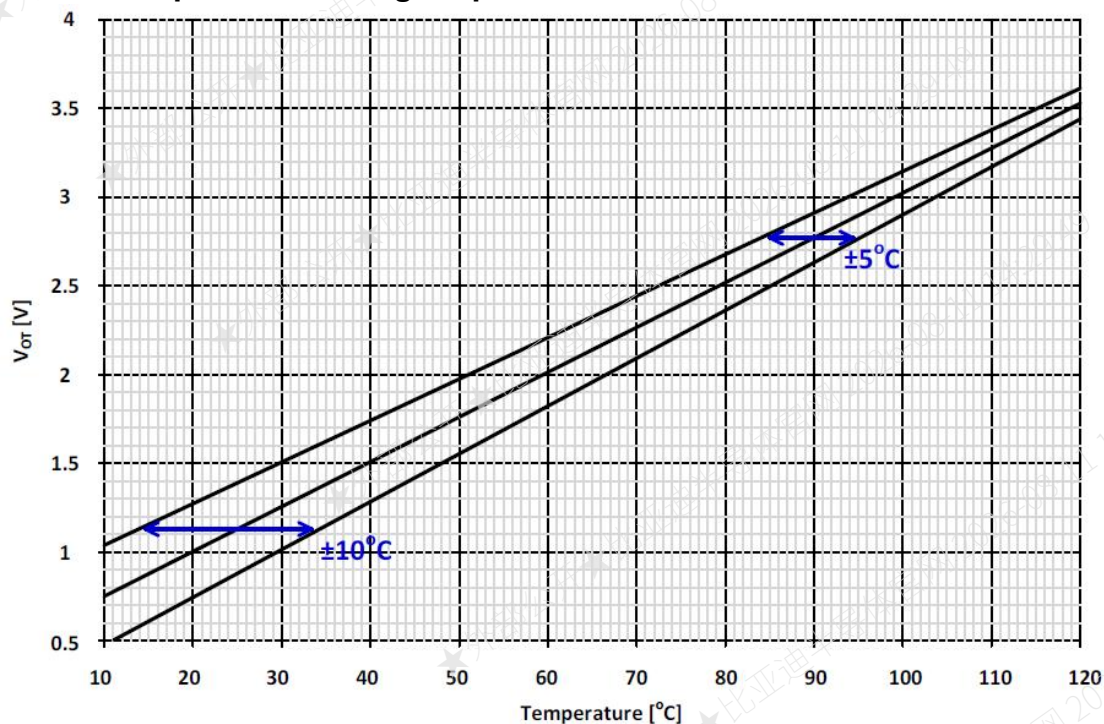
图 5. 温度输出电压 Fig 5. Voltage of temperature
