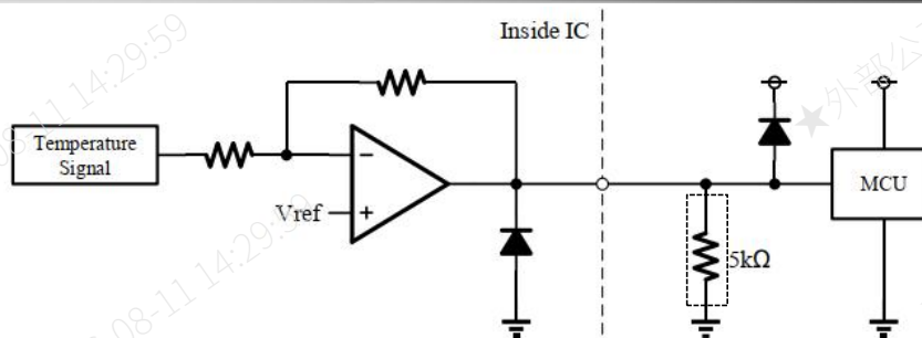
图 6. 温度输出电路 Fig 6. circuit of temperature
