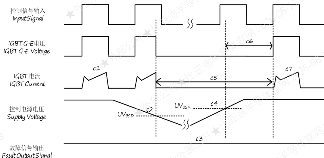
图 10. 上桥欠压保护
