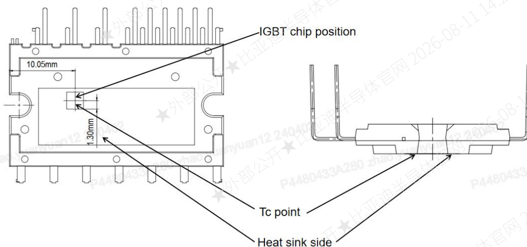
图 3. 壳温测试点 Fig 3. Tc Measurement Point
