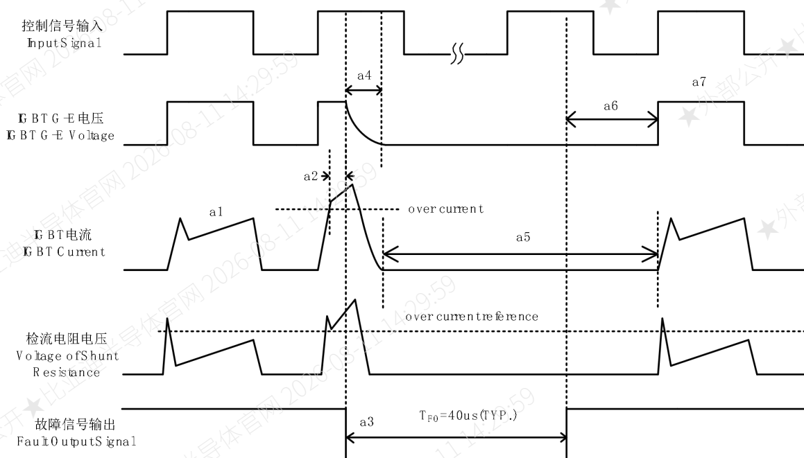
图 8. 过流保护 Fig 8. Over Current Protection
