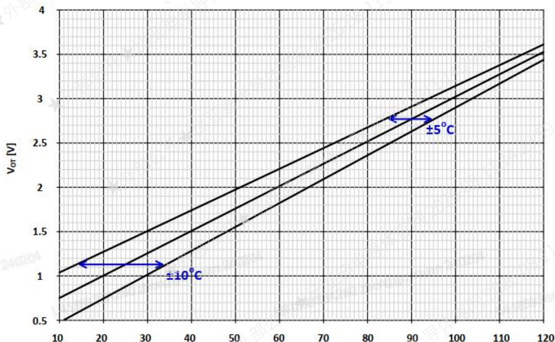
图 5. 温度输出电压
