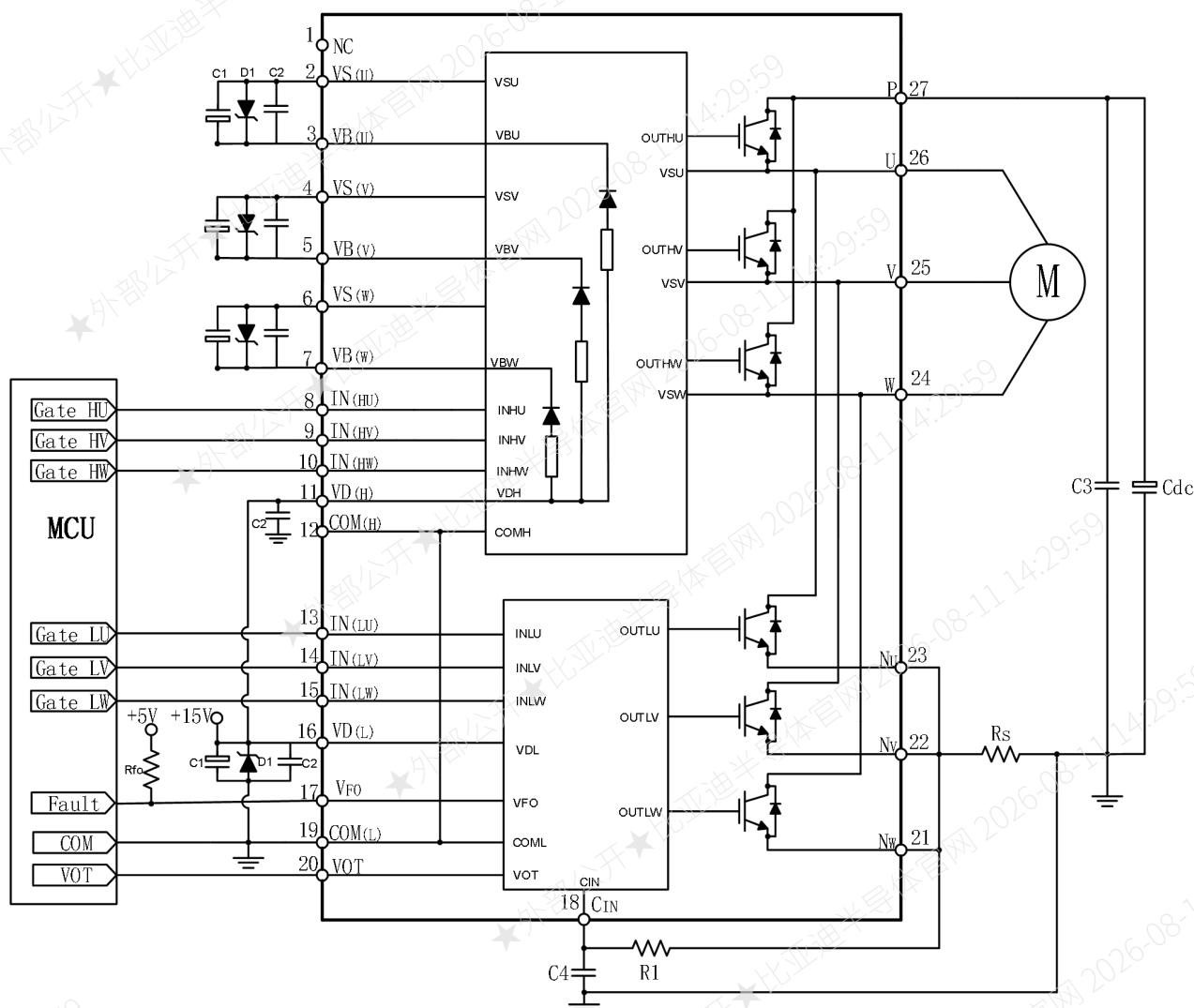
图 11. 典型应用电路 Fig 11. Typical Application Circuit
