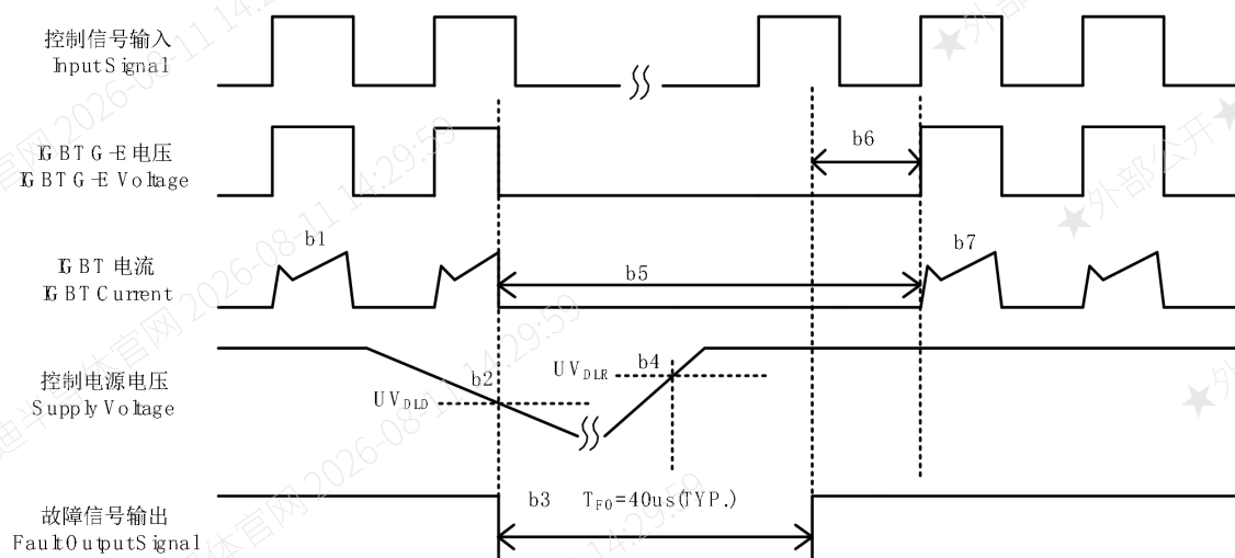
图 9. 下桥欠压保护
