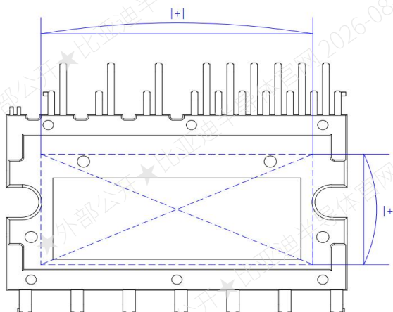
图 7. 平面度测量位置 Fig 7. Flatness Measurement Position
