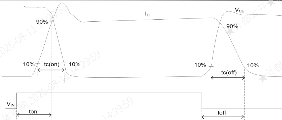
图 4. 开关时间定义 Fig 4. Switching Time Definition
