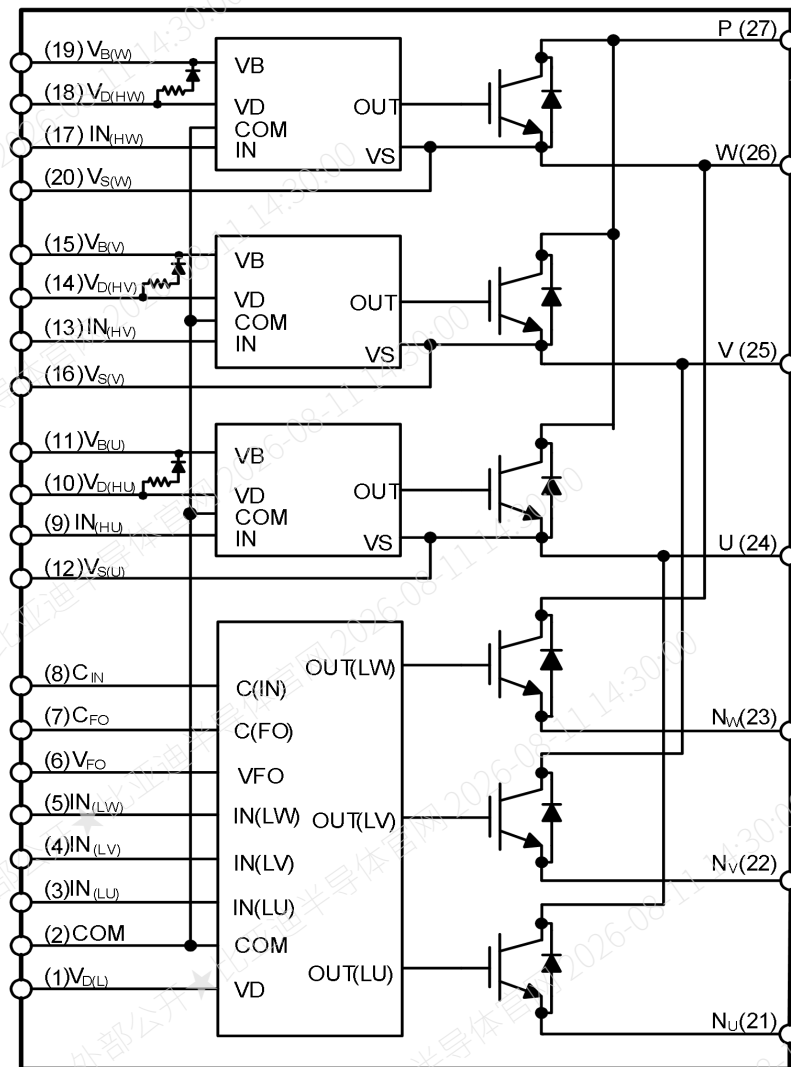
图 2. 内部等效电路和输入输出引脚 Fig 2. Internal Equivalent Circuit and Input/Output Pins
