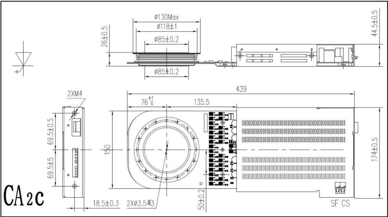
图7. IGBT器件外形图（单位：mm）
