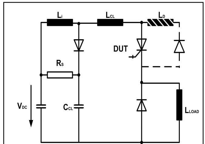
图13. RB_IGCT器件测试电路图
