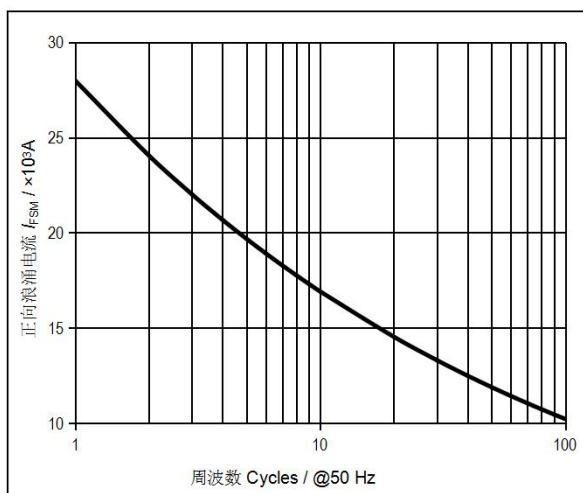
图5. 浪涌电流与周波数的关系曲线 Fig.5 Surge current vs cycles
