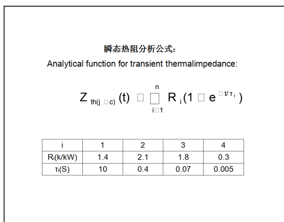
图9. 瞬态热阻抗分析公式
