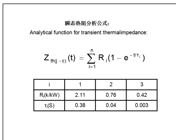
图3. 瞬态热阻抗分析算公式 Fig.3 Analytical function for transient thermal impedance
