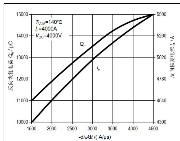
图4. 反向恢复电荷、电流与 di_F/dt 的关系曲线 Fig.4 Reverse recovery charge and current vs di_F/dt
