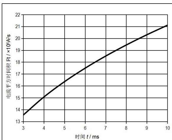
图7. I^2t 特性曲线 Fig.7 I^2t vs time
