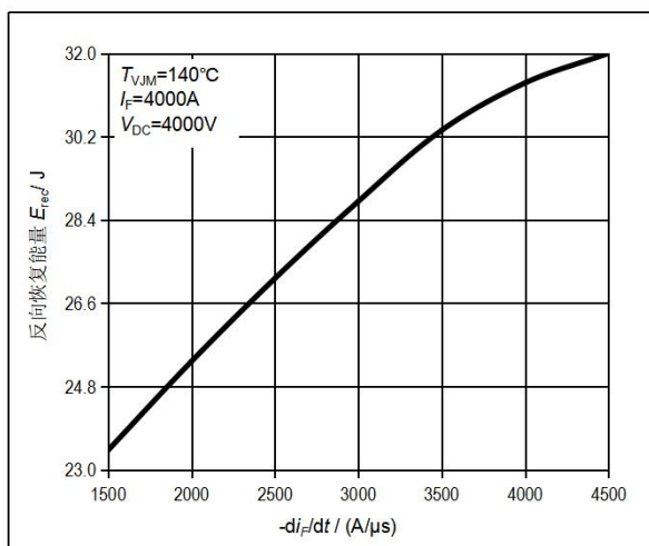
图5. 反向恢复能量与 di_F/dt 的关系曲线 Fig.5 Reverse recovery energy vs di_F/dt
