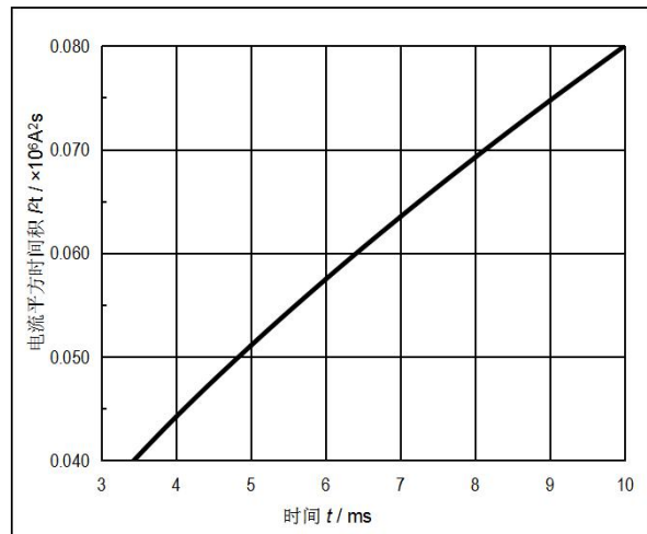
图6. I^2t 特性曲线 Fig.6 I^2t vs time
