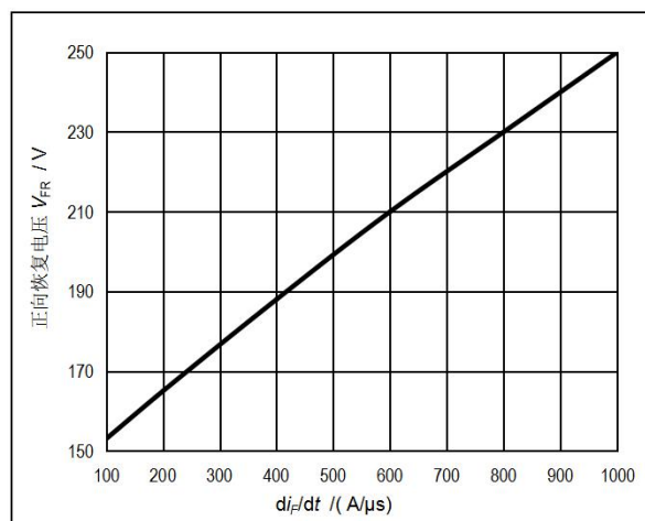
图3. 正向恢复电压与 di_F/dt 的关系曲线 Fig.3 Peak forward recovery voltage vs di_F/dt
