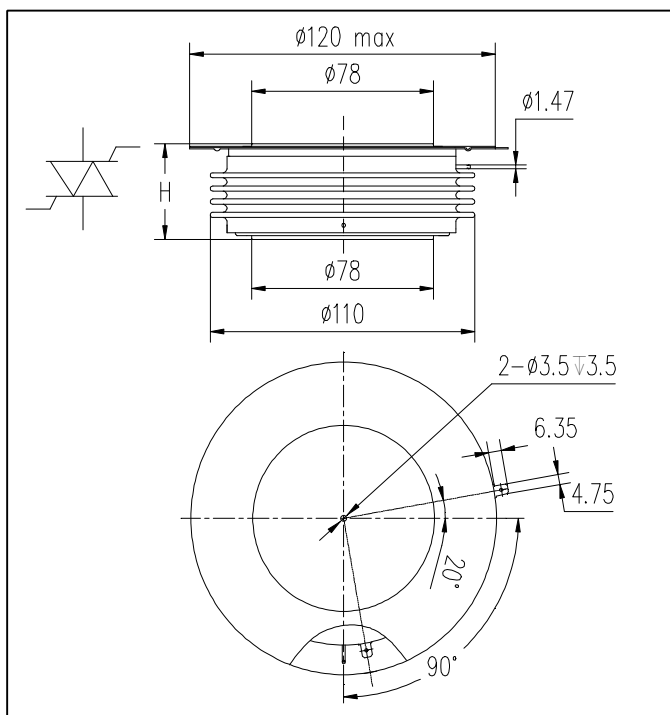
外形图 Outline
