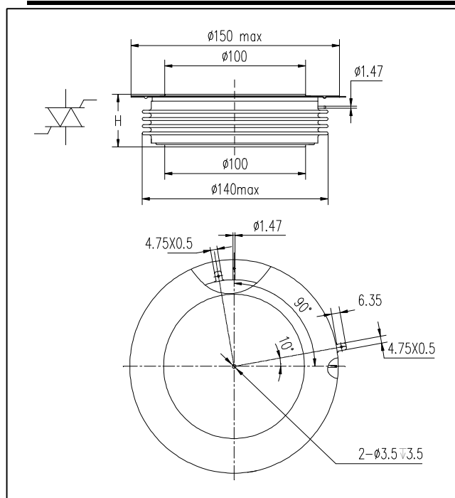
外形图 Outline
