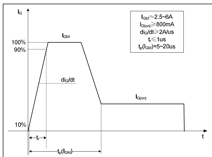
图9. 推荐门极触发波形
