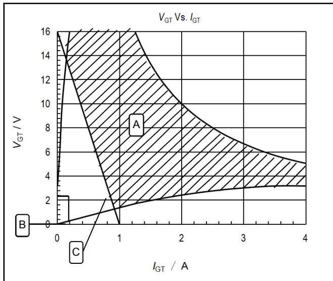
图8. 门极触发电特性曲线
