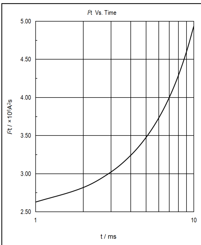
图6. I^2t 特性曲线
