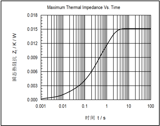
图2. 瞬态热阻曲线及分析曲线
