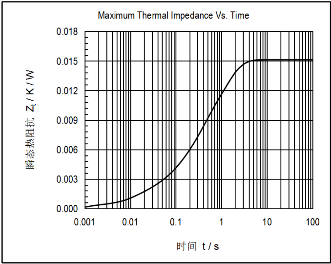
图2. 瞬态热阻曲线及分析公式
