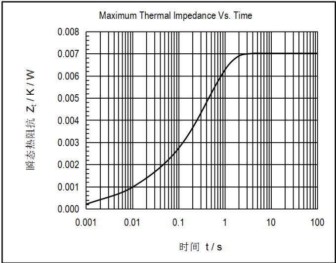
图3. 瞬态热阻抗曲线及分析公式
