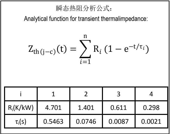
图3. 瞬态热阻抗曲线及分析公式
