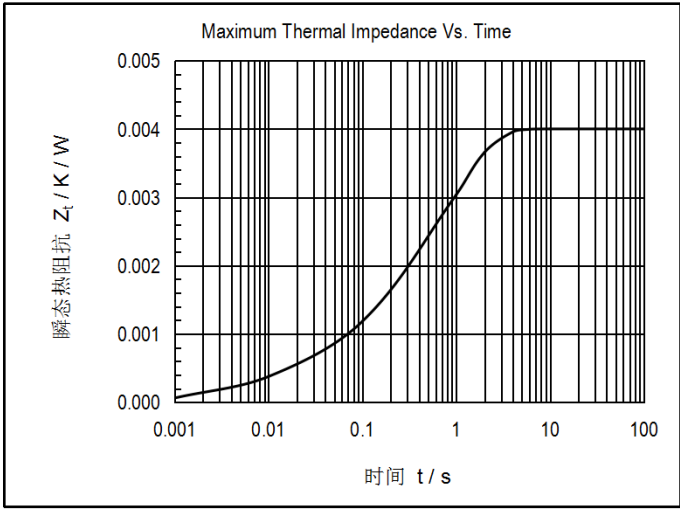
图2. 瞬态热阻抗曲线及分析曲线
