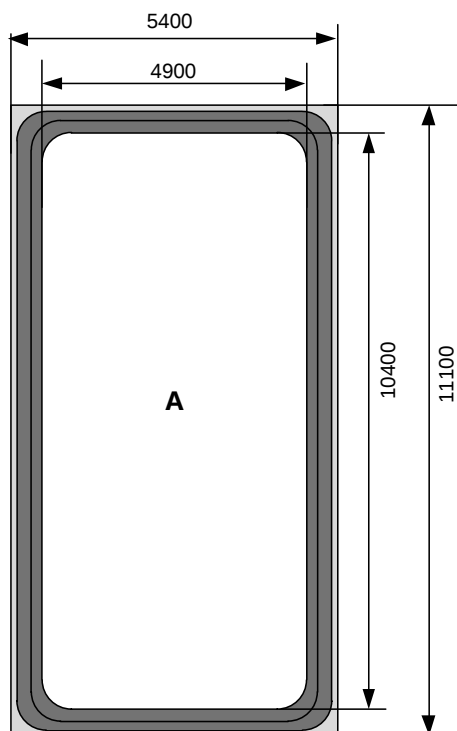
图 2. 芯片外观尺寸
