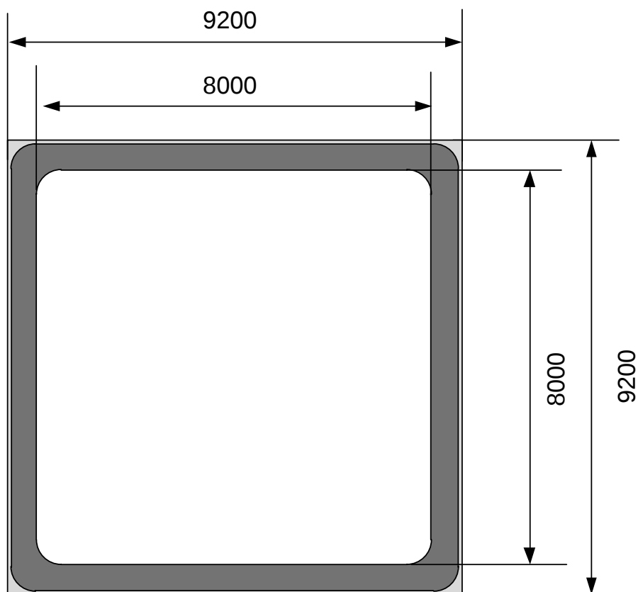
图 2. 芯片外观尺寸
