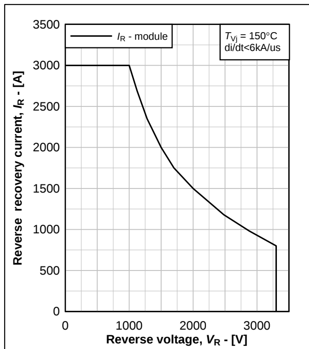
图 8. 二极管反偏安全工作区, I_R = f(V_R)
