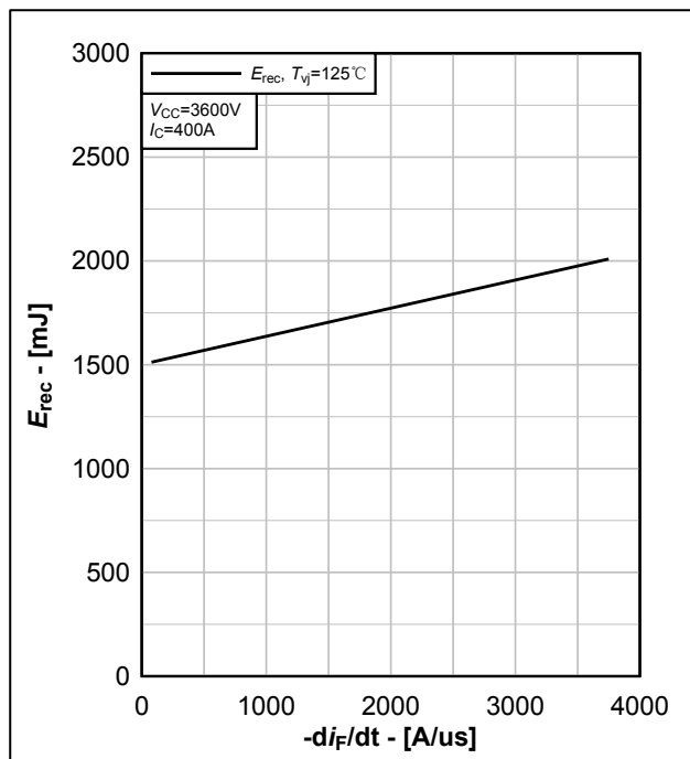
图 5.反向恢复损耗典型曲线, E_{rec} = f(-di_F/dt)
