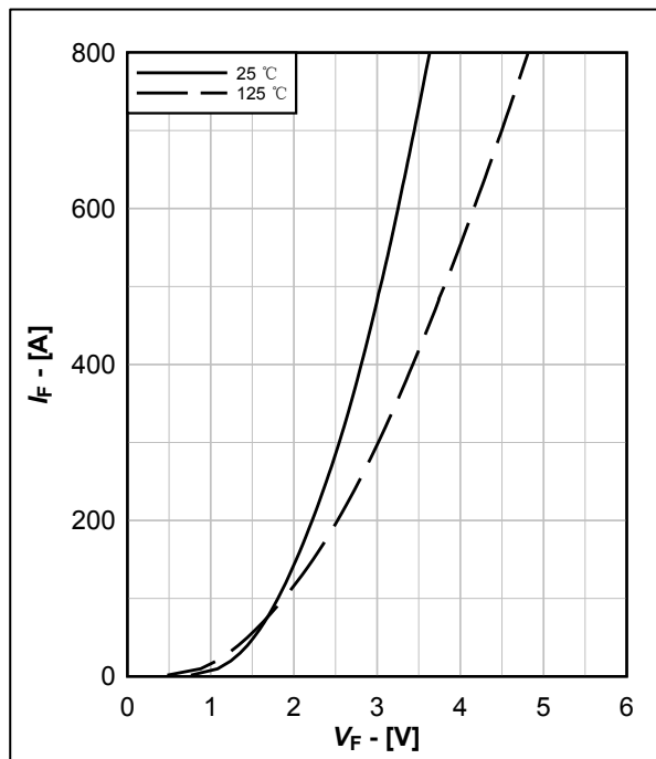
图 3.输出特性典型曲线, I_F = f(V_F)
