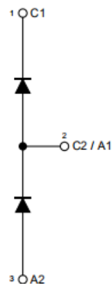
图 1.电路结构
