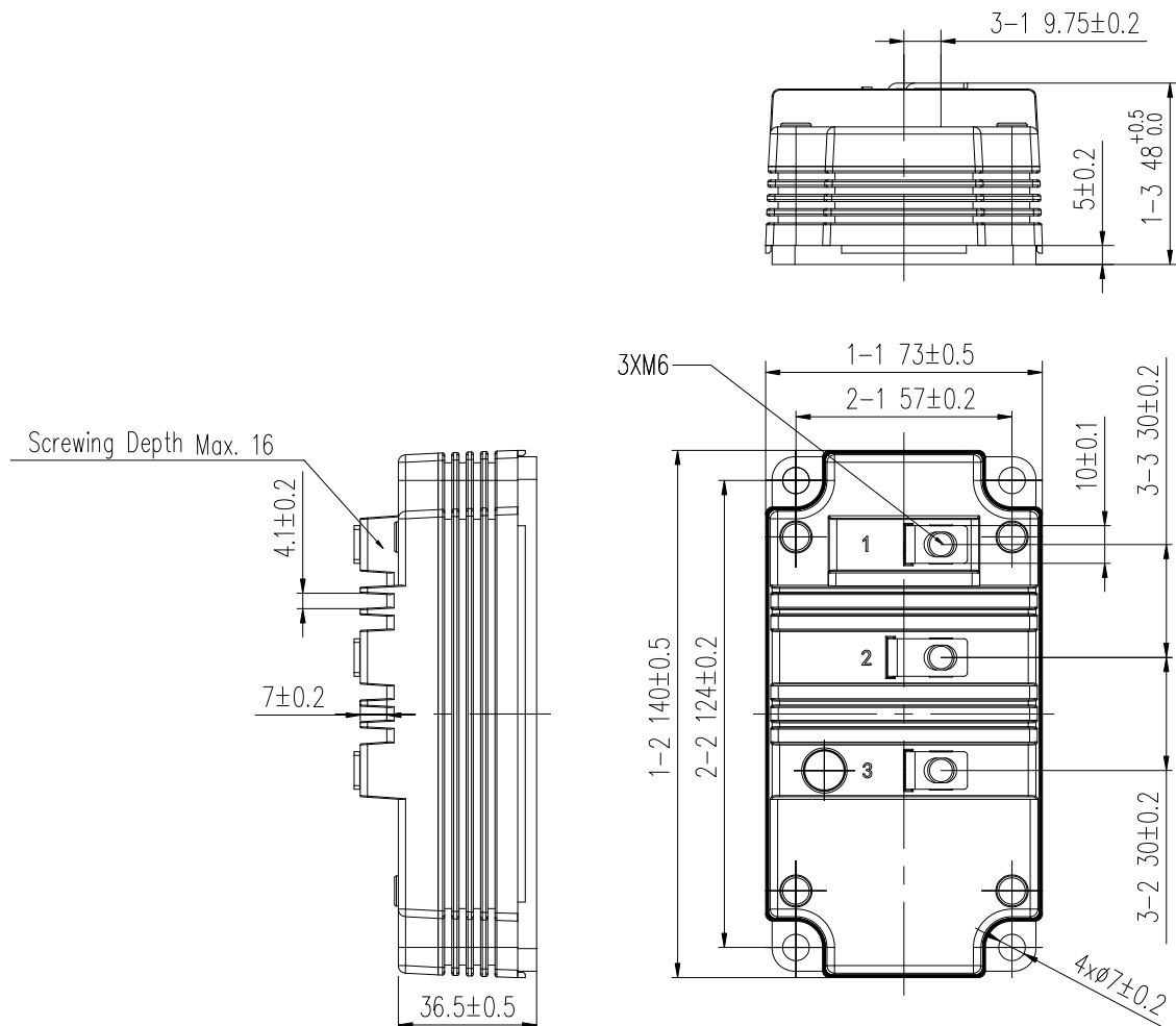
图 10. 模块外观尺寸
