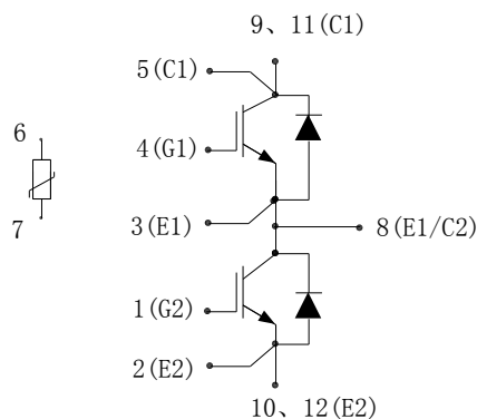
图 1. 电路结构
