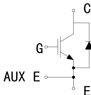
图 1. 电路结构
