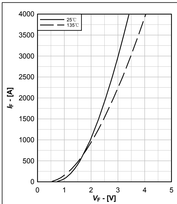
图 8. FRD 输出特性典型曲线, I_F = f(V_F)
