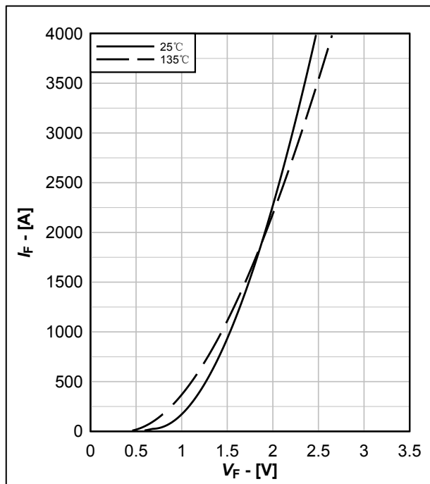
图 8. FRD 输出特性典型曲线, I_F = f(V_F)
