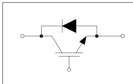
图 1. 电路结构
