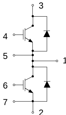
图 1. 电路结构
