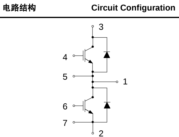
图 1. 电路结构
