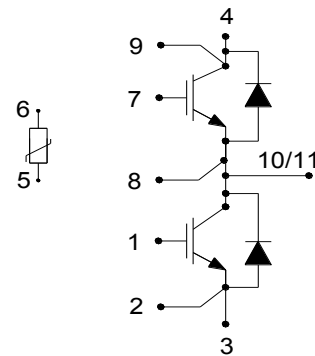
图 1. 电路结构
