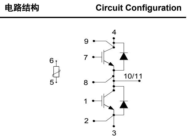
图 1. 电路结构
