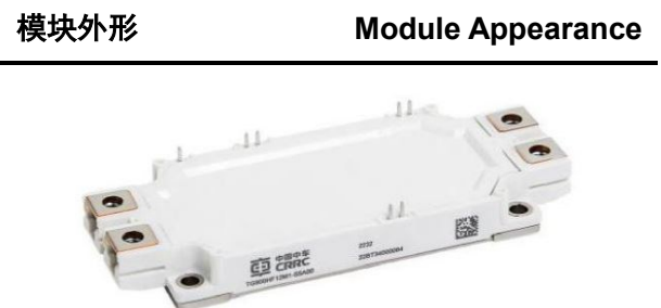
图 2. 模块外形
