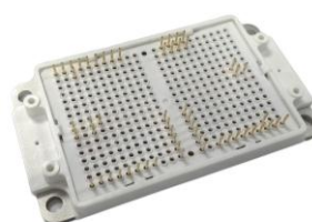
图 2. 模块外形
