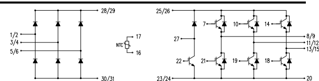
图 1. 电路结构
