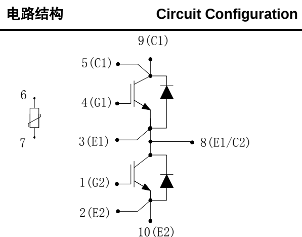
图 1. 电路结构
